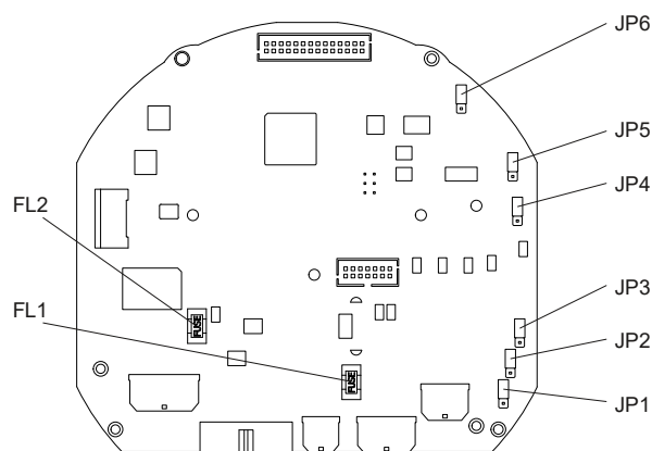
Bild 77: Logikplatine
