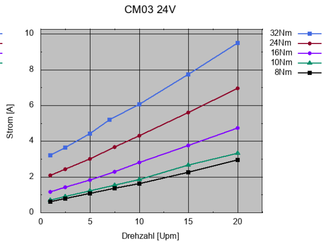
Bild 93: Stromaufnahme der 24 VDC-Version
