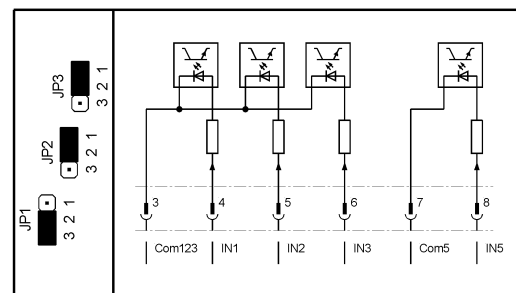
Bild 82: 3 Eingänge mit gemeinsamer Masse und ein getrennter Eingang. Der Eingang IN4 ist deaktiviert.
