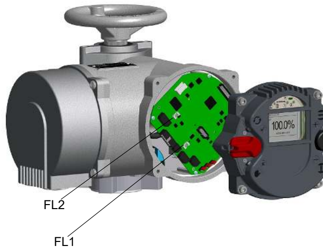
Bild 75: FL1... Sicherung für die Hilfsspannung, FL2... Sicherung für die binären Ausgänge
