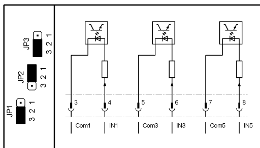
Bild 81: Drei getrennte Eingänge Die Eingänge IN2 und IN4 sind deaktiviert.
