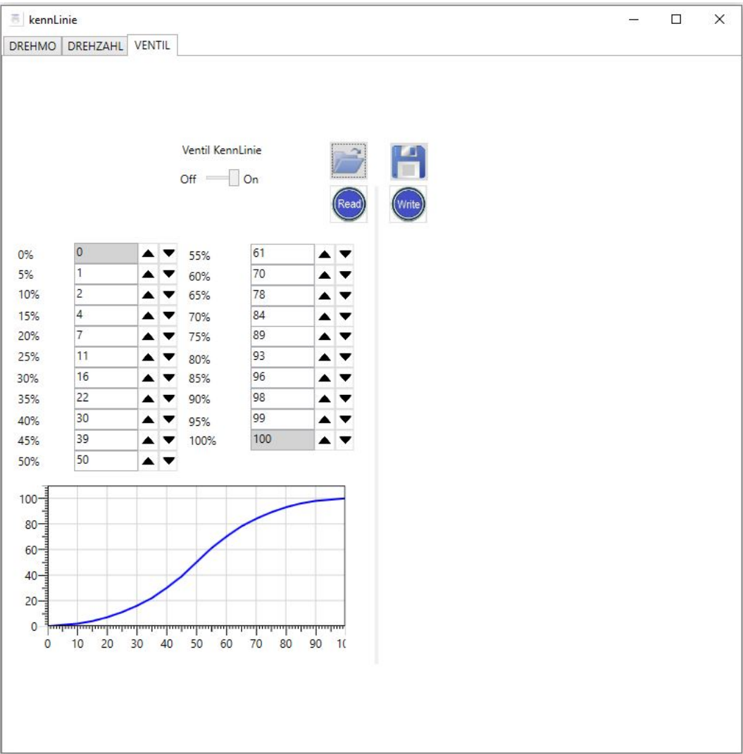
Bild 64: Ventil Kennlinie
