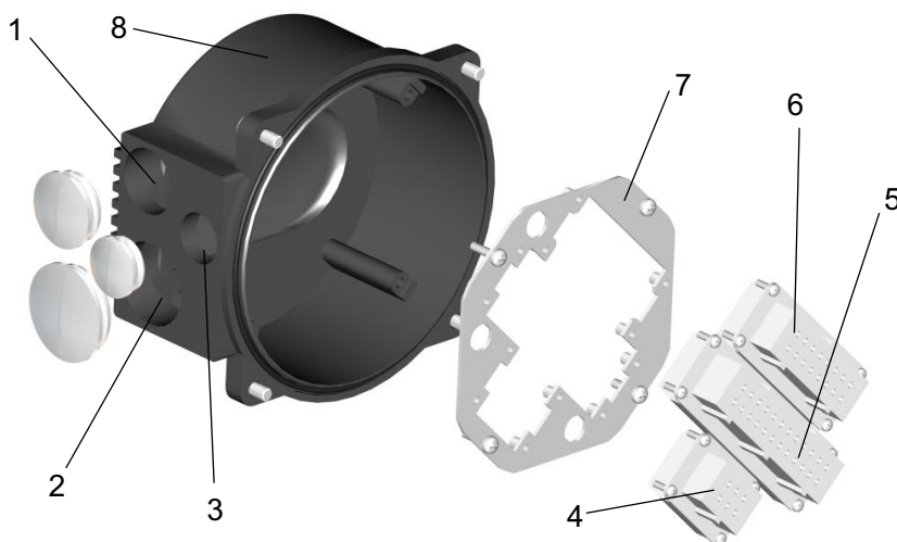
Bild 11: 1... Metrische Verschraubung M32x1,5, 2... M40x1,5, 3... M25x1,5, 4... Steckereinsatz Han6E (für Spannungsversorgung), 5... Steckereinsatz Han24E (für Steuerleitungen), 6... Stecker für Optionen, 7... Steckerblech, 8... Anschlussgehäuse
