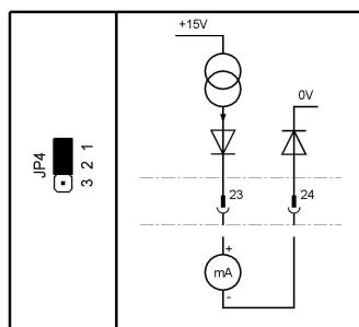
Bild 90: Stromquelle (aktiver mA-Ausgang)
