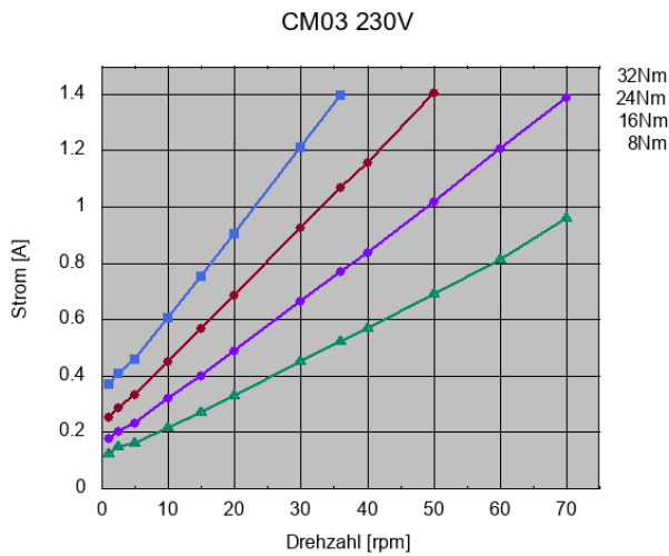
Bild 92: Stromaufnahme der Standard-Version
