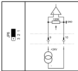
Bild 88: Passiver Eingang (Standard)
