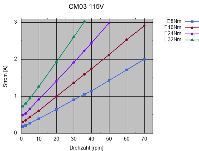
Bild 94: Stromaufnahme der Standard-Version
