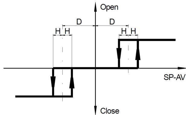
Bild 61: Funktionsweise der Totzone und der Hysterese bei den Zwischenstellungen
