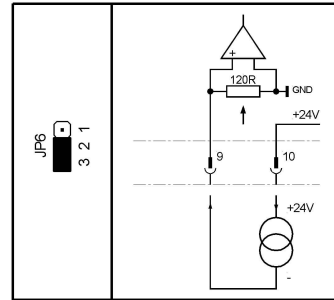
Bild 89: Eingang mit interner Versorgung (aktiver Eingang)
