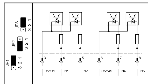
Bild 80: Je zwei Eingänge mit gemeinsamer Masse, beide Massen getrennt. Der Eingang IN3 ist deaktiviert.
