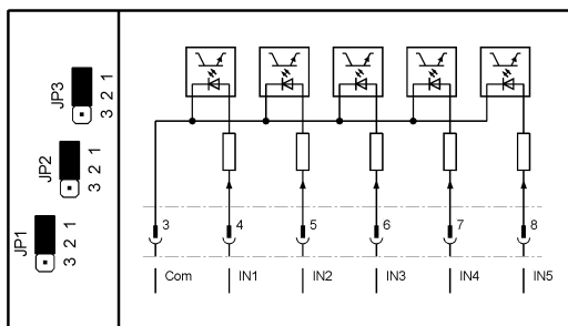
Bild 79: 5 Eingänge mit gemeinsamer Masse
