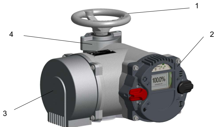
Bild 1: 1... Handrad, 2... Steuerung (Bedieneinheit), 3... Anschlussraum 4... Getriebeteil
