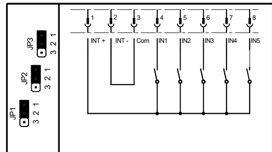
Bild 85: 5 Eingänge mit gemeinsamen "-" und interner 24V Spannung (z.B. potentialfreie Kontakte)
