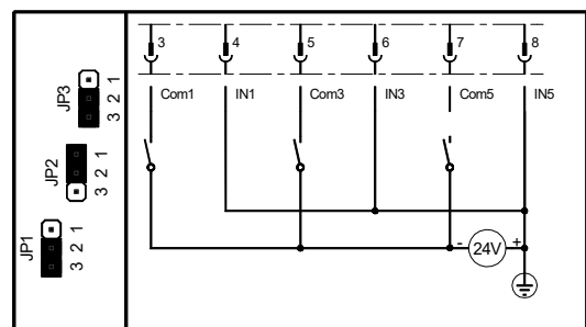
Bild 87: 3 getrennte Eingänge mit gemeinsamen "+" und externer 24V Spannung
