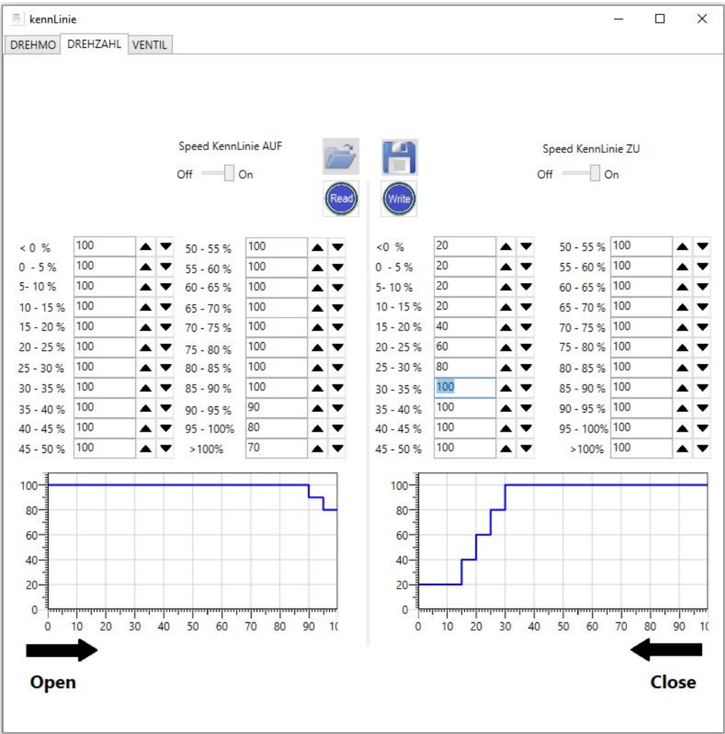
Bild 63: Drehzahl Kennlinie
