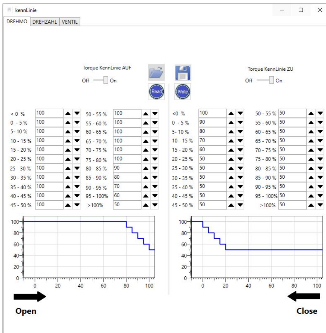
Bild 62: Drehmoment Kennlinie
