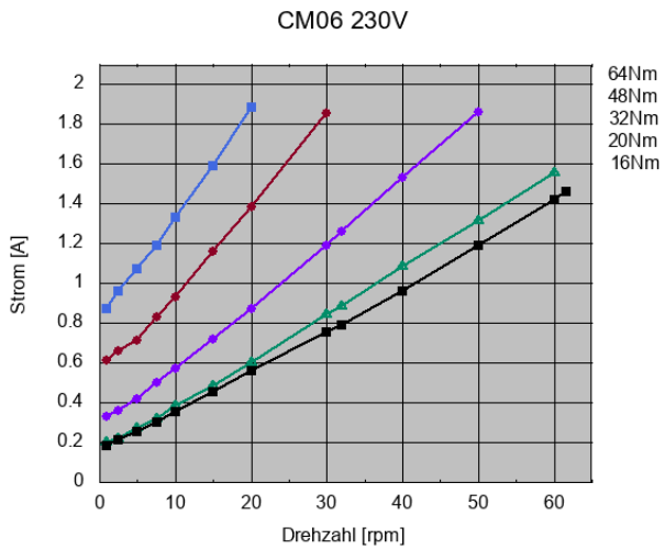
Bild 95: Stromaufnahme der Standard-Version
